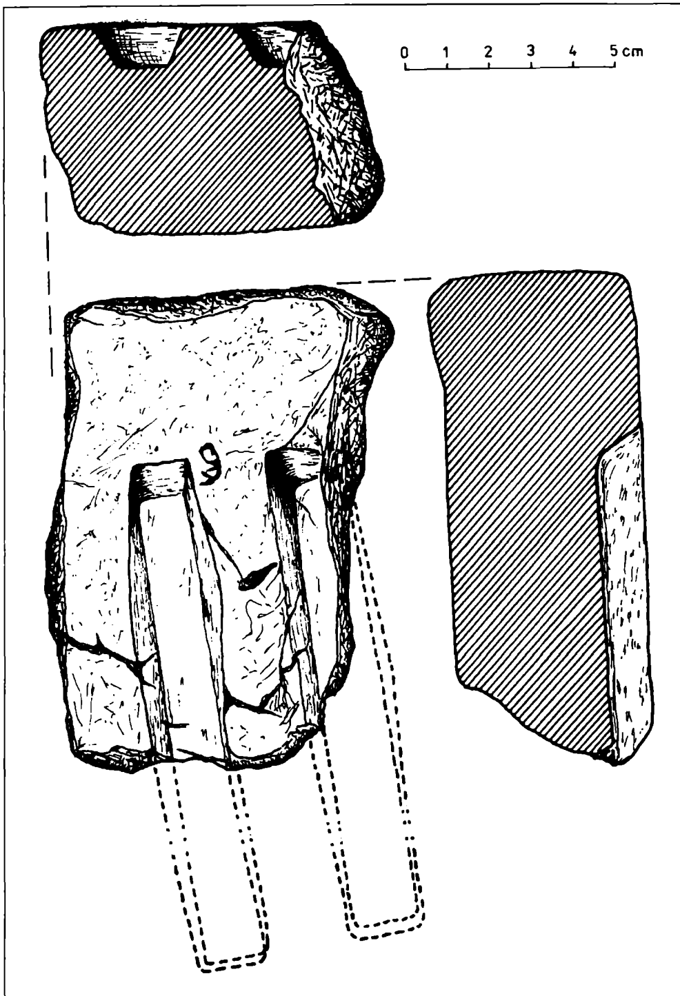
Fig. 1 Tiparul fragmentar pentru turnat lingouri de metal
